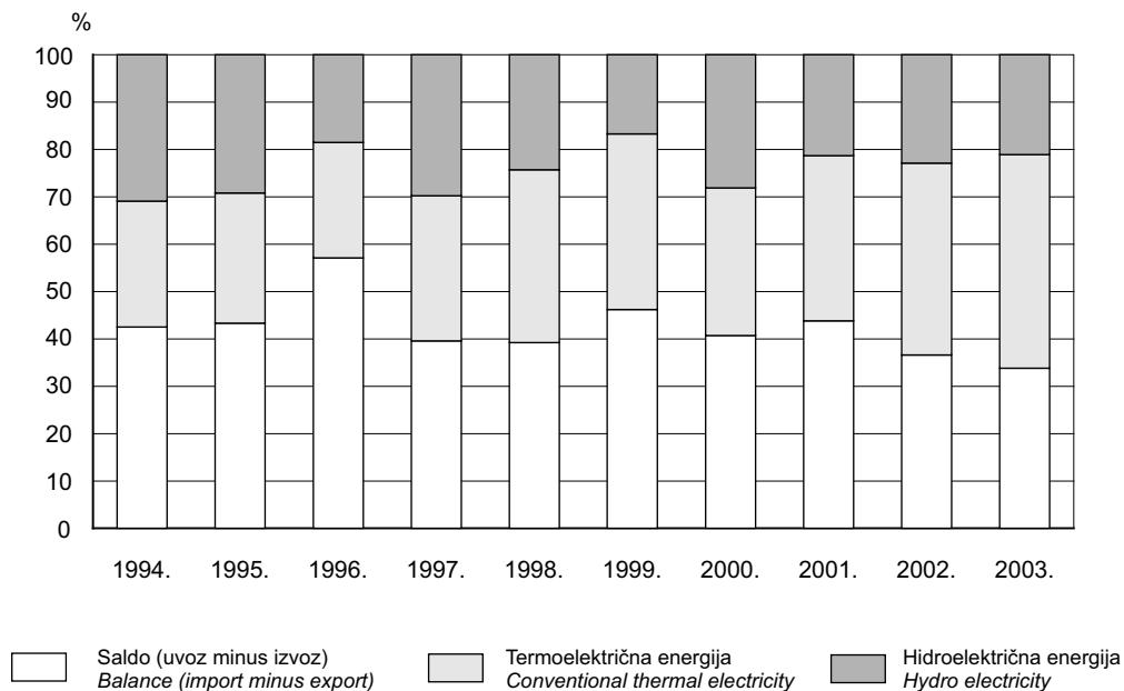
G 19-1. STRUKTURA RASPOLOŽIVE ELEKTRIČNE ENERGIJE OD 1994. DO 2003. STRUCTURE OF ELECTRICITY AVAILABLE FOR INTERNAL MARKET 1994 – 2003
