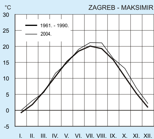
G 1-1. GODIŠNJI HOD TEMPERATURE ZRAKA U 2004. I ZA RAZDOBLJE OD 1961. DO 1990. ANNUAL AIR TEMPERATURE CHANGE, 2004 AND 1961 - 1990
