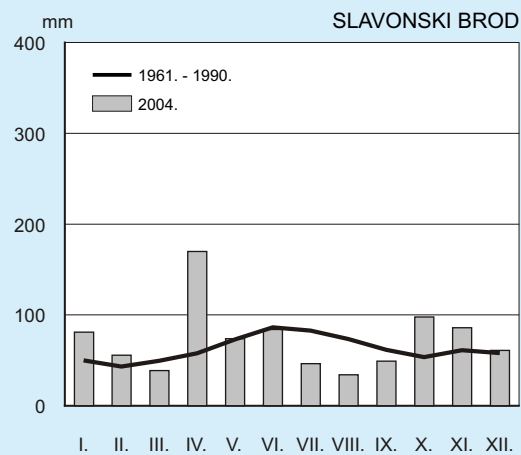
G 1-2. GODIŠNJI HOD KOLIČINE OBORINA ZA 2004. I ZA RAZDOBLJE OD 1961. DO 1990. ANNUAL PRECIPITATION CHANGE, 2004 AND 1961 - 1990
